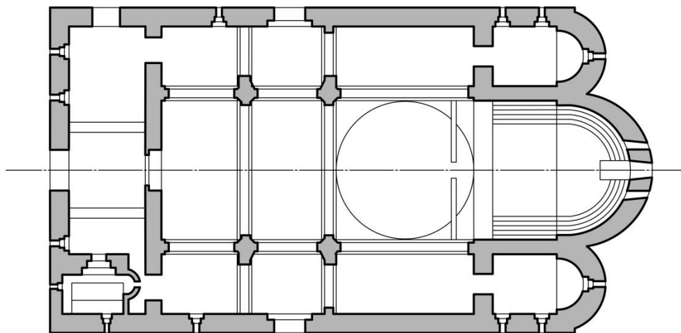
Рис. 5. План храма № 8. Пицунда
