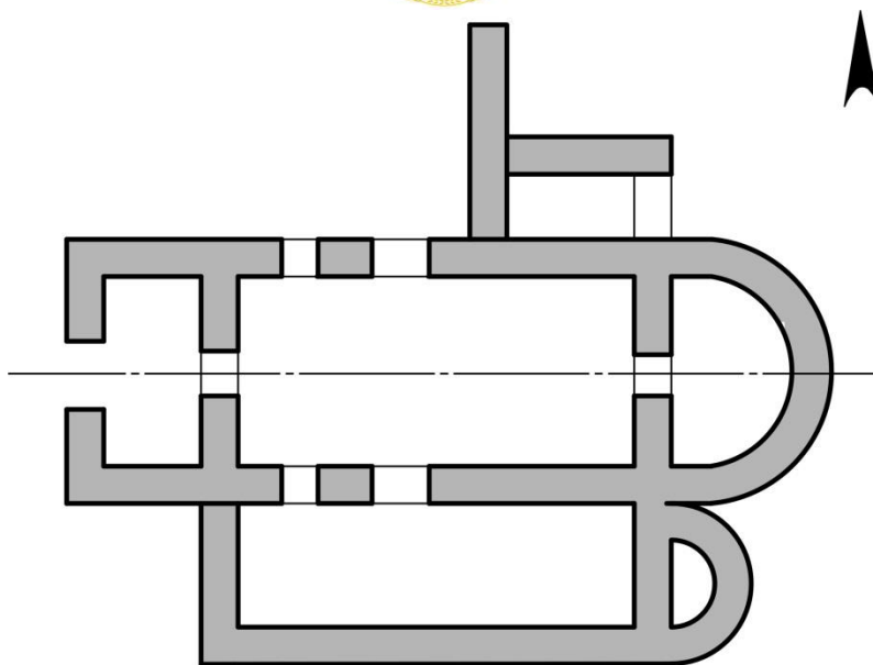
Рис. 9. План базилики Леснянской № 2
