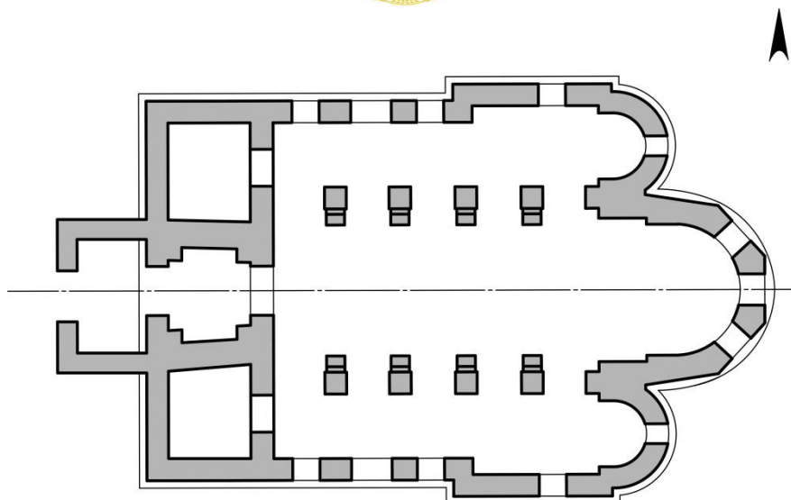
Рис. 3. План Цандрипшской базилики
