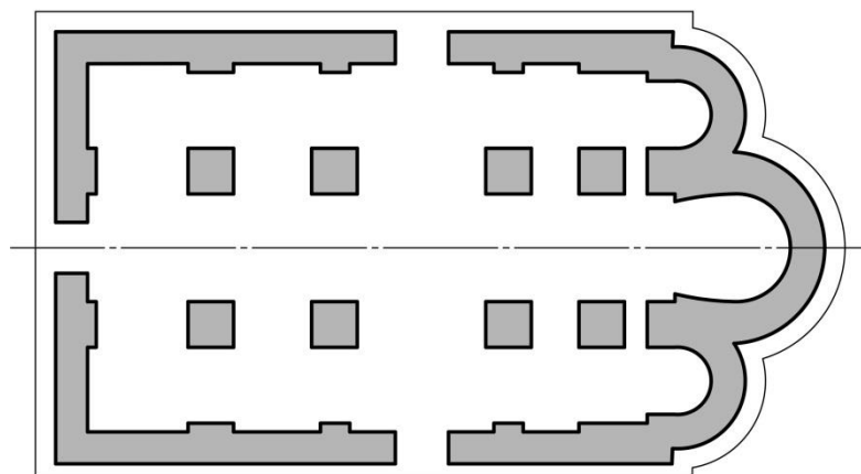
Рис. 6. План храма № 3. Алахадзы
