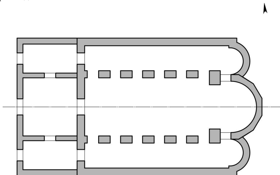
Рис. 4. План храма № 1. Алахадзы
