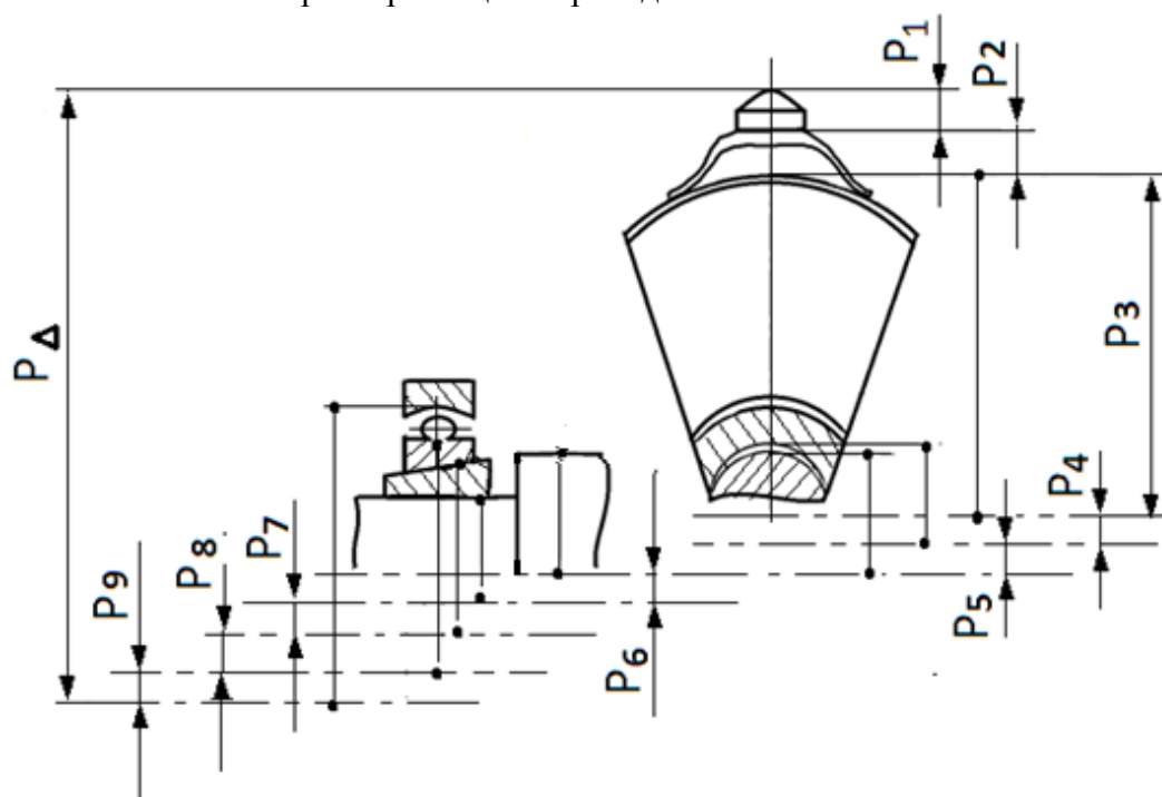
Рис. 1. Размерная цепь формирования радиуса расположения вершин рабочего профиля бичей
