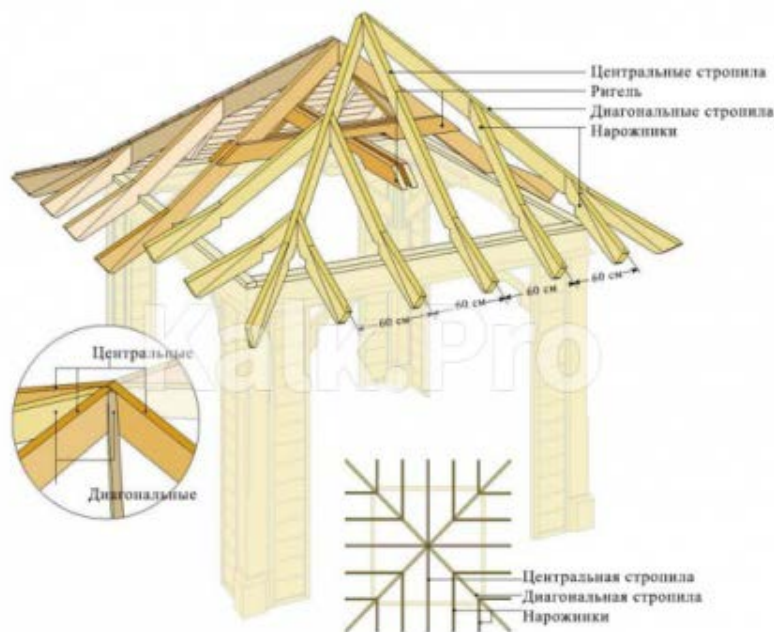
Рис. 5. Шатровая кровля
