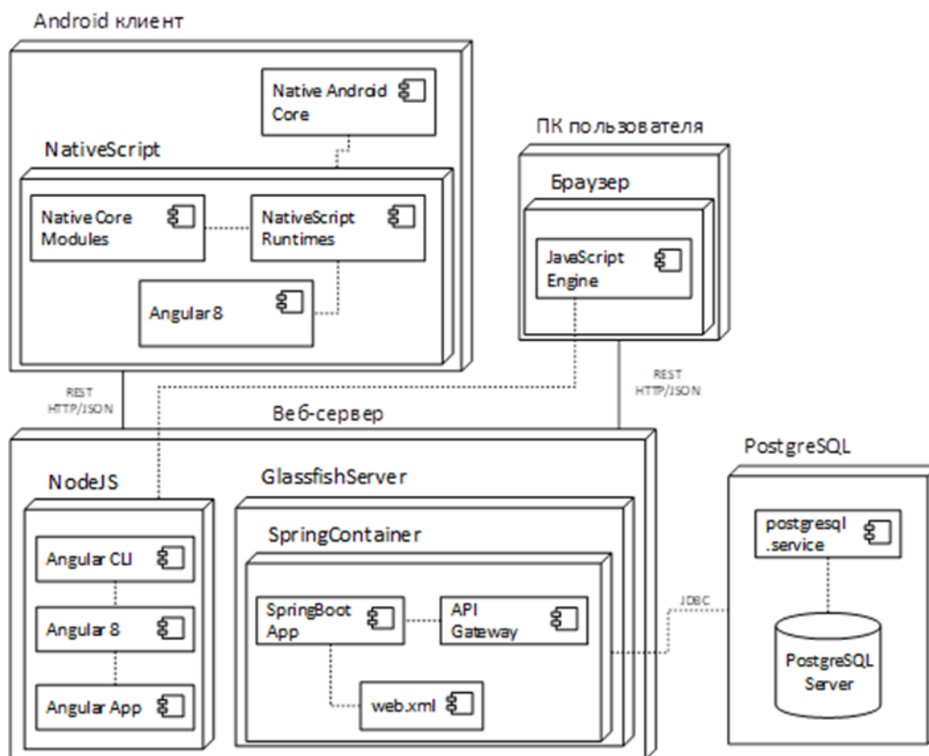
Рис. 1. Диаграмма развертывания приложения на Angular 8
