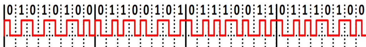
Рис. 2. Сообщение Test в манчестерском кодировании
