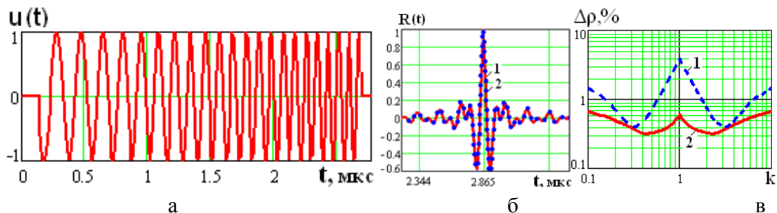
Рис. 2. Обработка линейно-частотно-модулированного радиоимпульса
