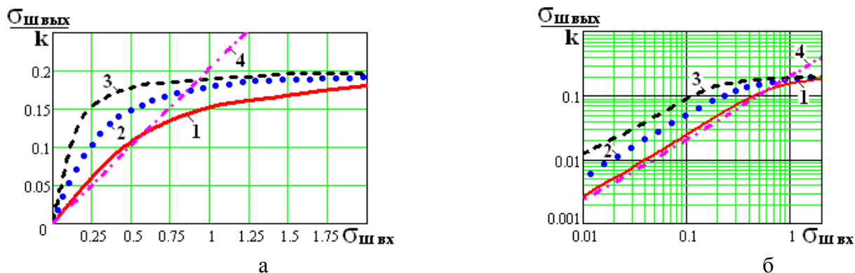
Рис. 4. Зависимости СКО выходного шума
