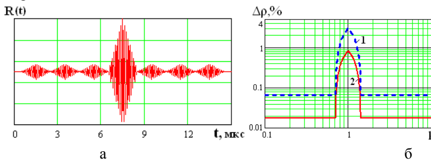
Рис. 1. Обработка фазоманипулированного радиоимпульса
