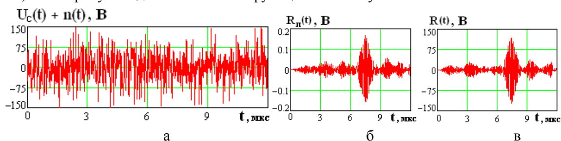
Рис. 5. Входные и выходные сигналы согласованных фильтров
