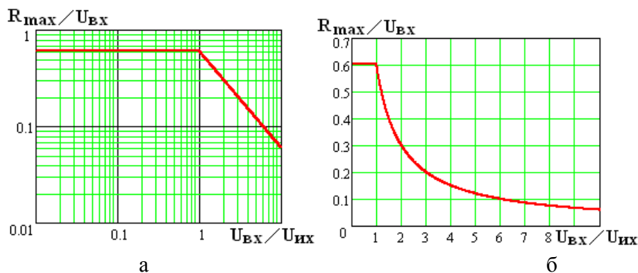
Рис. 3. Амплитудные характеристики СФ ФМИ
