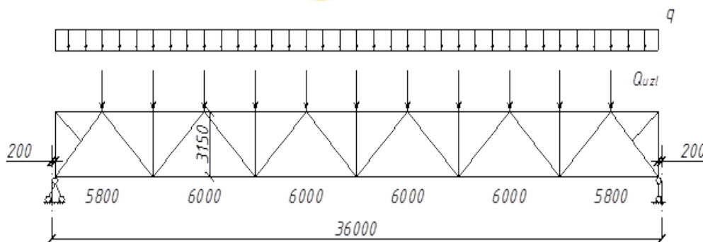
Рис. 1. Расчётная схема стропильной фермы
