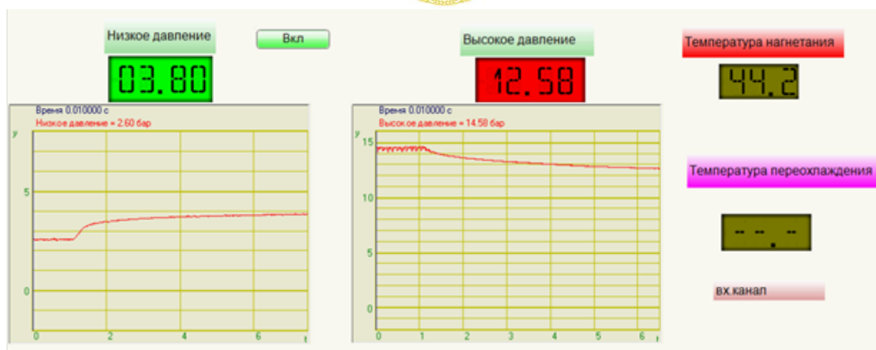
Рис. 3. Показания давлений на момент выключения установки, работающей в тяжелых условиях эксплуатации
