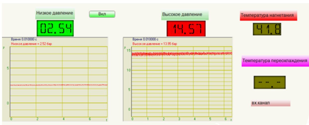
Рис. 4. Показания давлений на электродвигателе и на муфте компрессора кондиционера, работающего в тяжелых условиях эксплуатации
