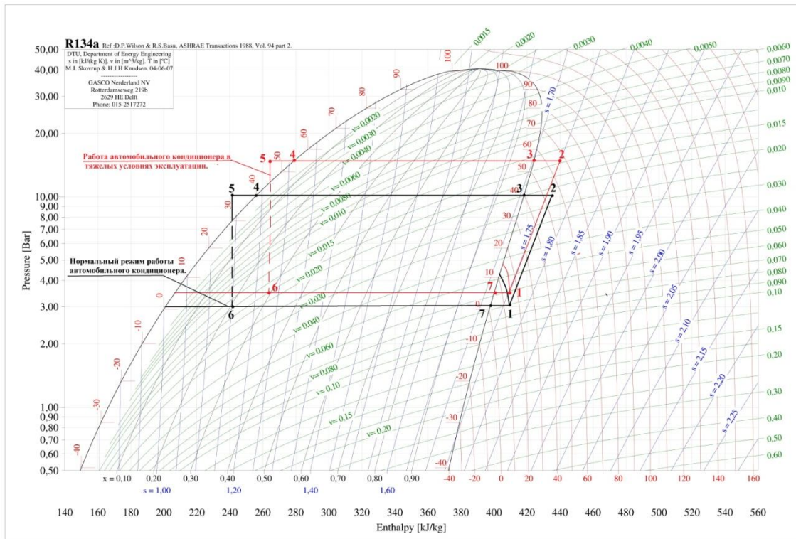
Рис. 5. Циклы холодильной машины автомобильного кондиционера при нормальной работе и при работе в тяжелых условиях эксплуатации
